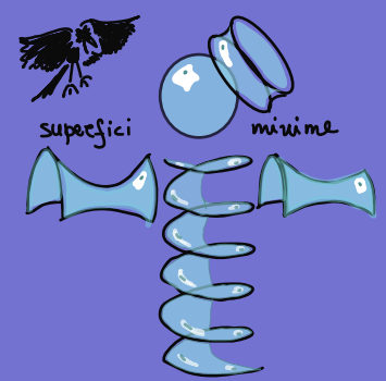
ANALISI GEOMETRICA
