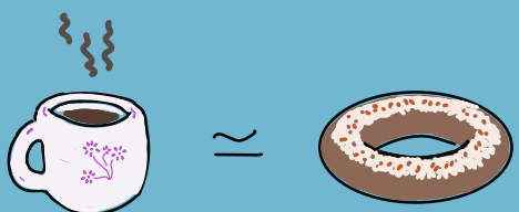
TOPOLOGIA ALGEBRICA
