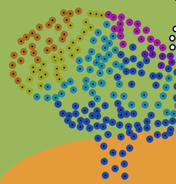
INTELLIGENZA ARTIFICIALE
