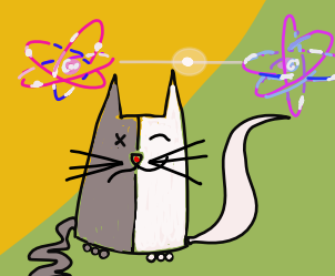
MECCANICA QUANTISTICA
