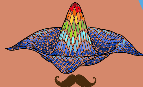
ANALISI NUMERICA
