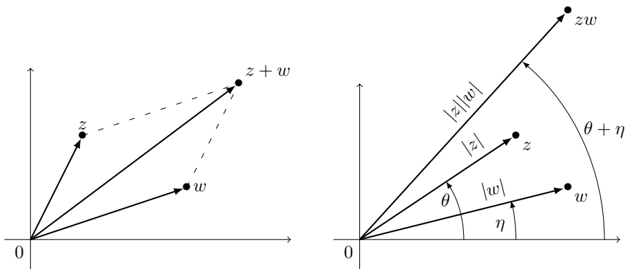
FIGURA 3.6. Rappresentazione geometrica di somma e prodotto; si noti come la disuguaglianza |z+w| \leq |z|+|w| equivale al fatto che in un triangolo la lunghezza di un lato non supera la somma delle lunghezze degli altri due.
