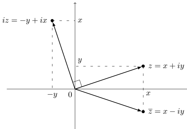
FIGURA 3.4. Geometricamente, il coniugato corrisponde alla riflessione rispetto all'asse reale e la moltiplicazione per l'unità immaginaria corrisponde alla rotazione di 90 gradi in senso antiorario.
