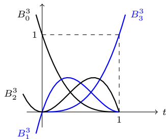
FIGURA 16.3. Grafici dei polinomi di Bernstein B_i^3(t) per 0 \leq t \leq 1 e 0 \leq i \leq 3 .
