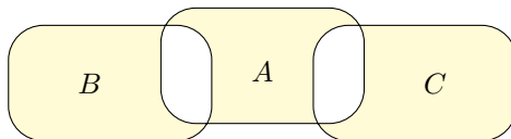
FIGURA 1.1. Visualizzazione grafica di A \cap (B \cup C) = (A \cap B) \cup (A \cap C) .
